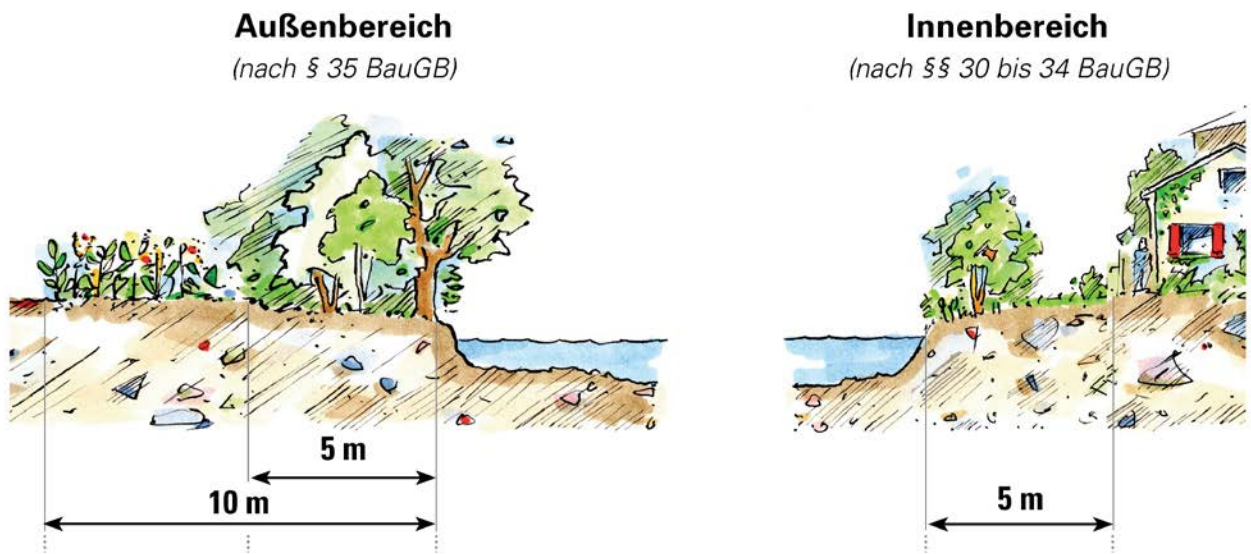
Bild 42: Ausdehnung des Gewässerrandstreifen gemäß § 29 Abs. 1 WG
