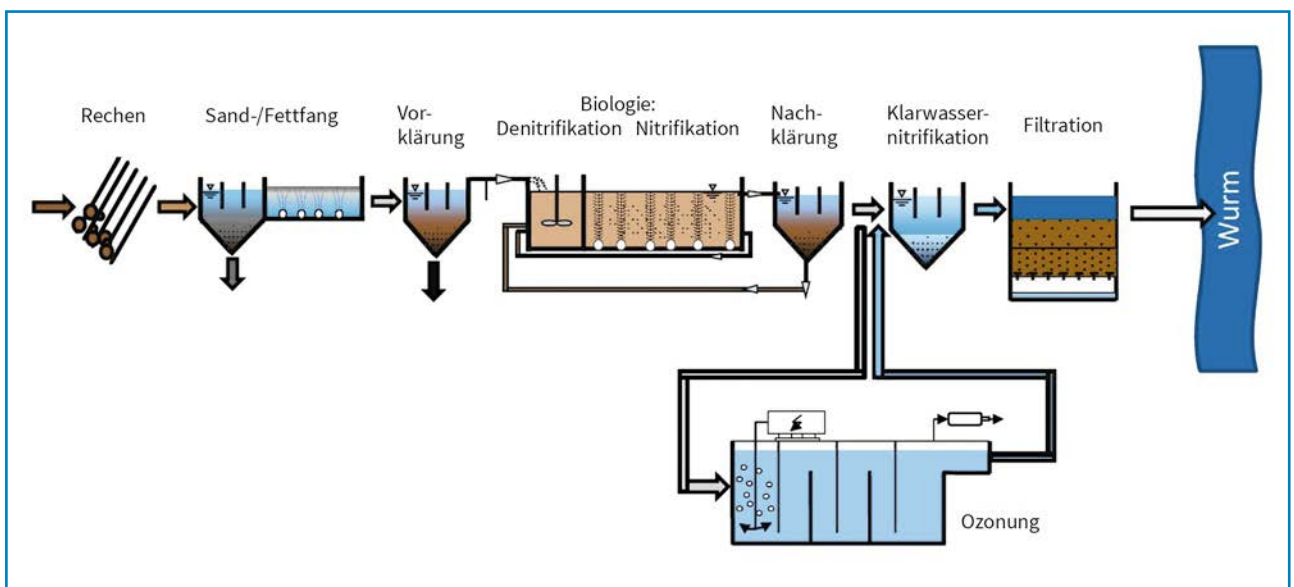
Bild 39: Verfahrensfliessbild der Kläranlage Aachen-Soers inkl. Ozonung
