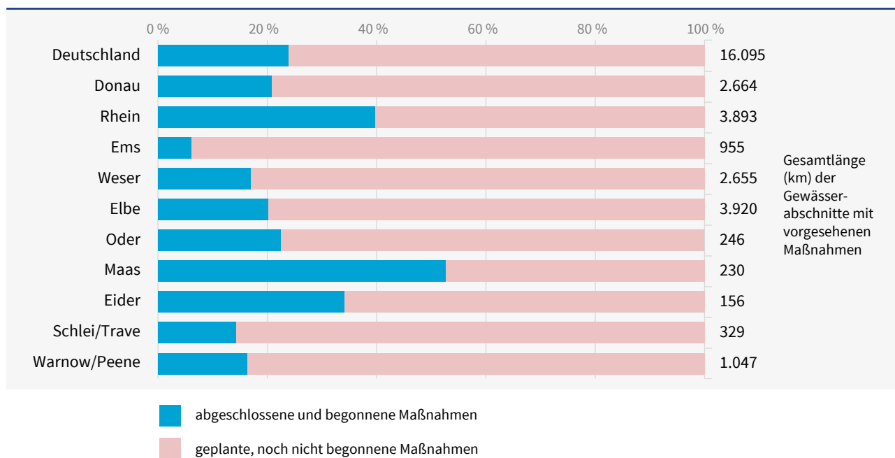
Abbildung 3-2: Umsetzungsstand der Maßnahmen zur Habitatverbesserung bezogen auf die Gesamtlänge der Gewässerabschnitte mit Maßnahmen (Datengrundlage: Angaben der Länder, Stand: Ende 2018)
