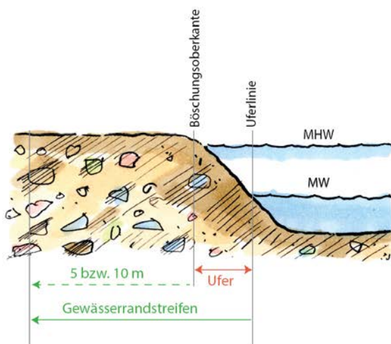
Bild 43: Bei Gewässern mit ausgeprägter Böschungsoberkante wird der Gewässerrandstreifen ab der Böschungsoberkante bemessen. (MW = Mittelwasser, MHW = mittleres Hochwasser)
